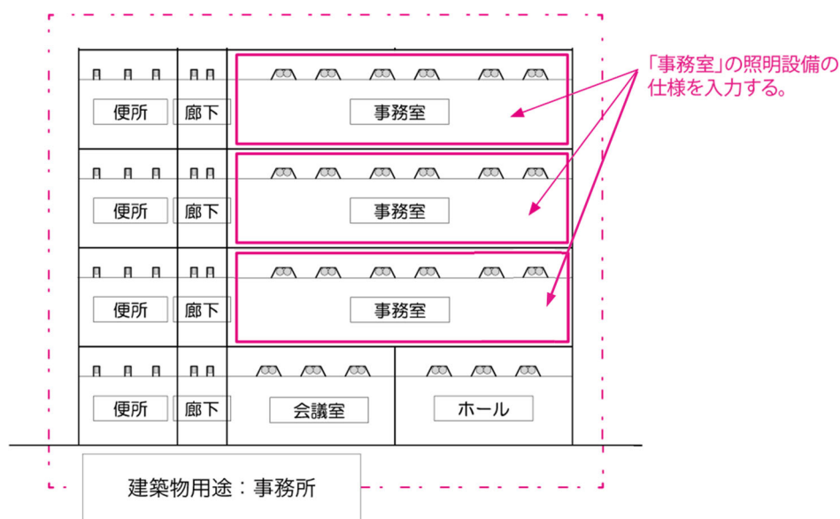
図 5-1-1 仕様を入力する照明設備の範囲（規模の小さな事務所の例）
