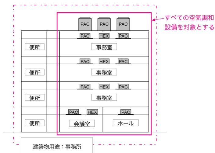
図 3-1-1 使用を入力する空気調和設備の範囲（規模の小さな事務所の例）
