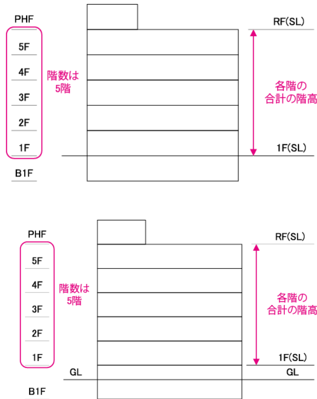
図 2-2-3 「各階の階高の合計」の算出方法（スラブレレベル間で算出する場合）
