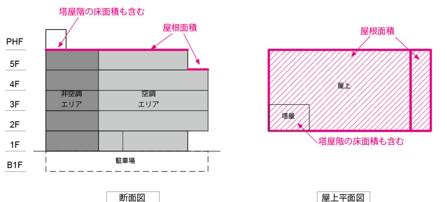
図 2-2-17 屋根面積の考え方
