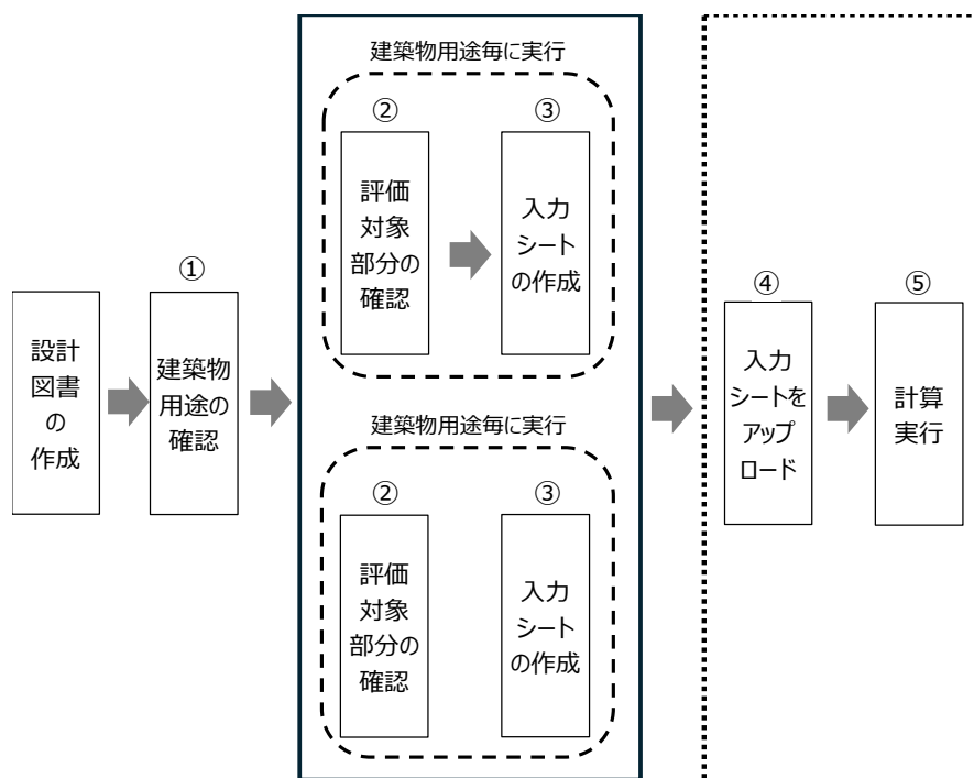
図 0-2-1 モデル建物法による評価の流れ
