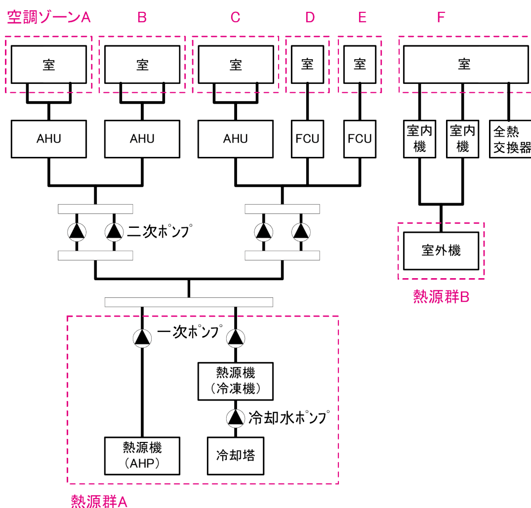
図2-5-1 熱源群の例
