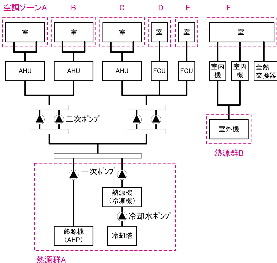
図2-5-1 熱源群の例
