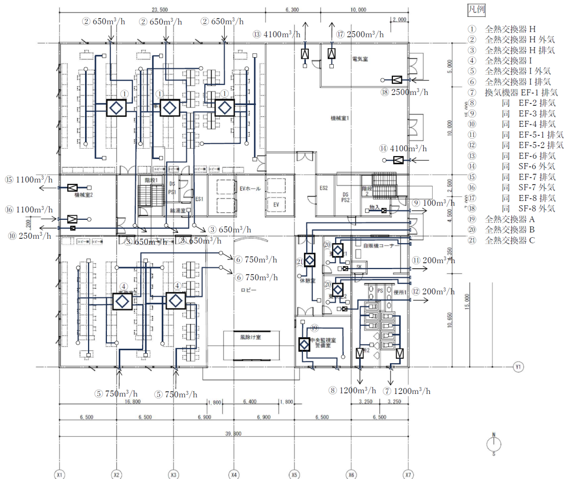
図 1 1 階の空調換気設備配置図及び各部風量（個別分散型空調設備の場合）
