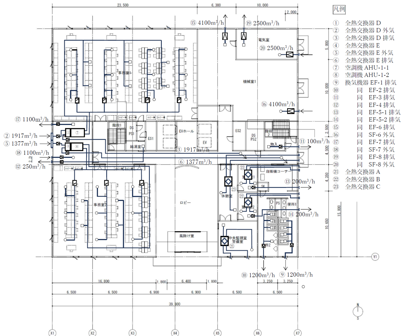
図3 1階の空調換気設備配置図及び各部風量（中央式空調設備）
