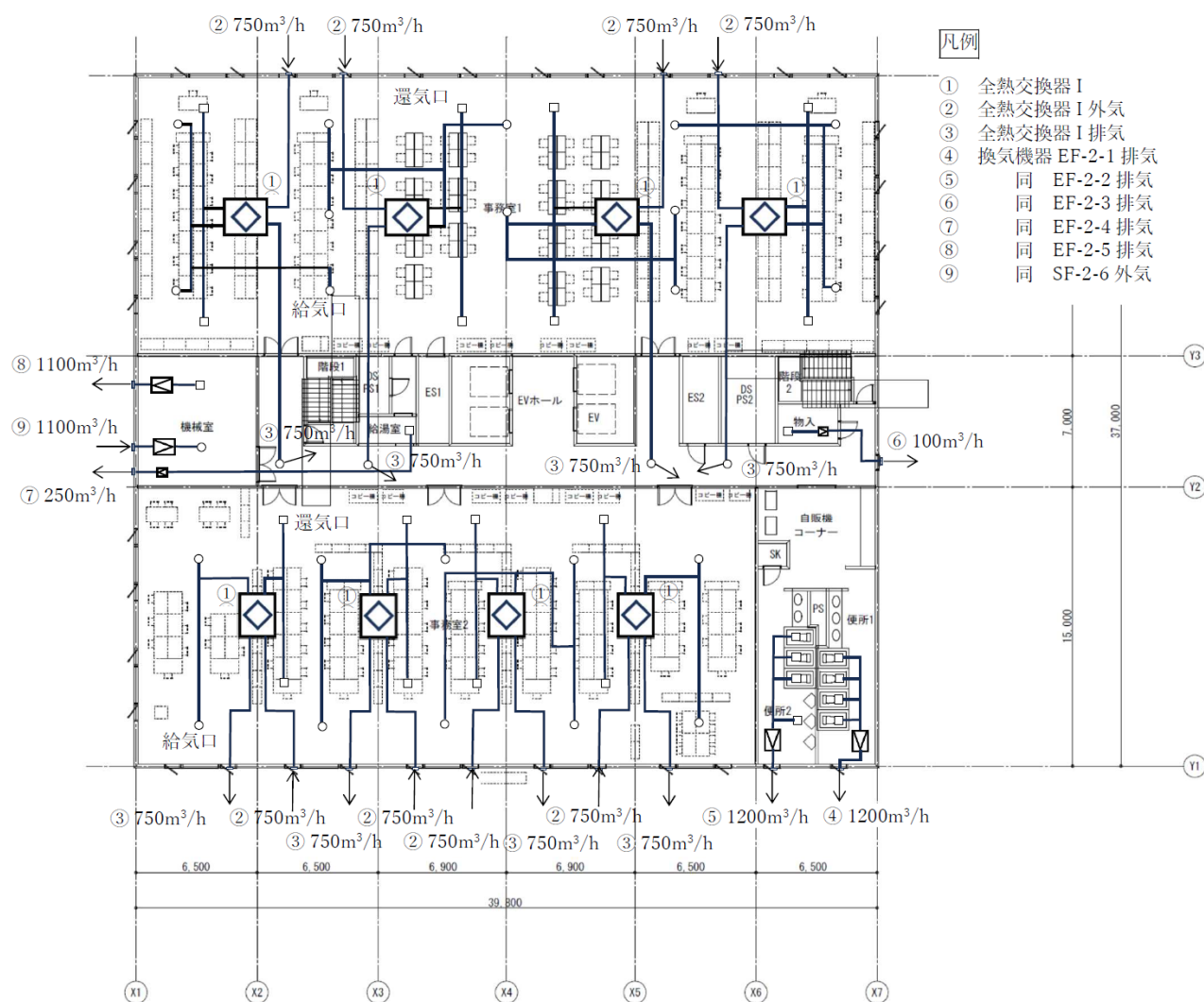
図2 標準階の空調換気設備配置図及び各部風量（個別分散型空調設備の場合）
