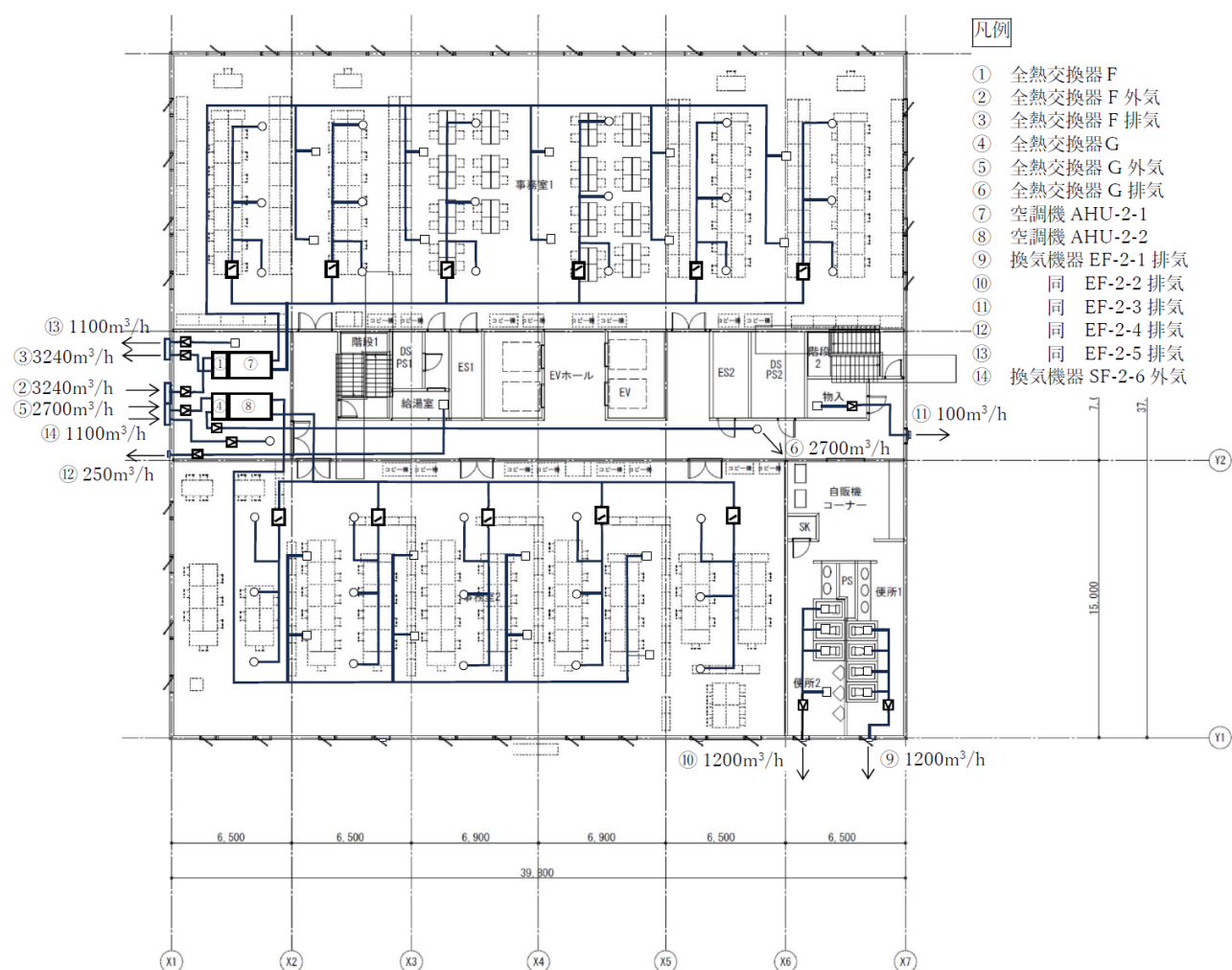
図4 標準階の空調換気設備配置図及び各部風量（中央式空調設備）
