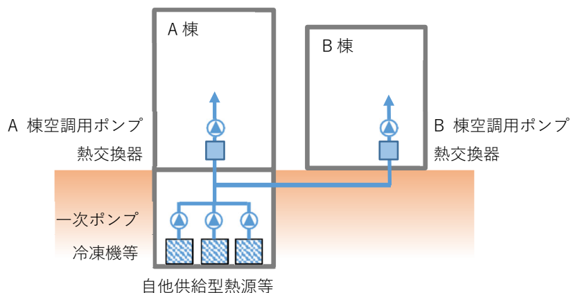
図 12-3-4 自他供給型熱源機器等が一次ポンプシステムの場合
