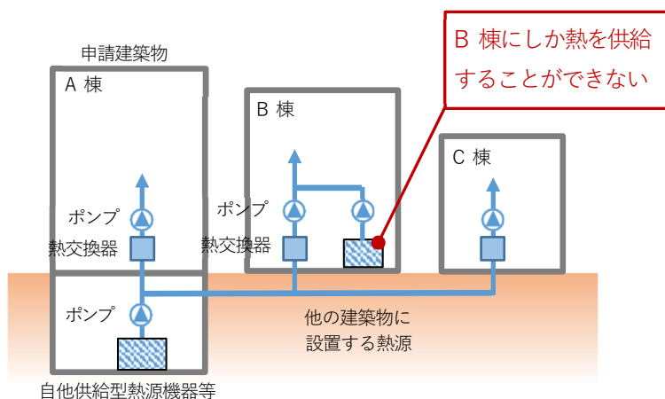
図 12-3-2 他の建築物に設置する熱源が、その建築物にのみ熱を供給する場合
