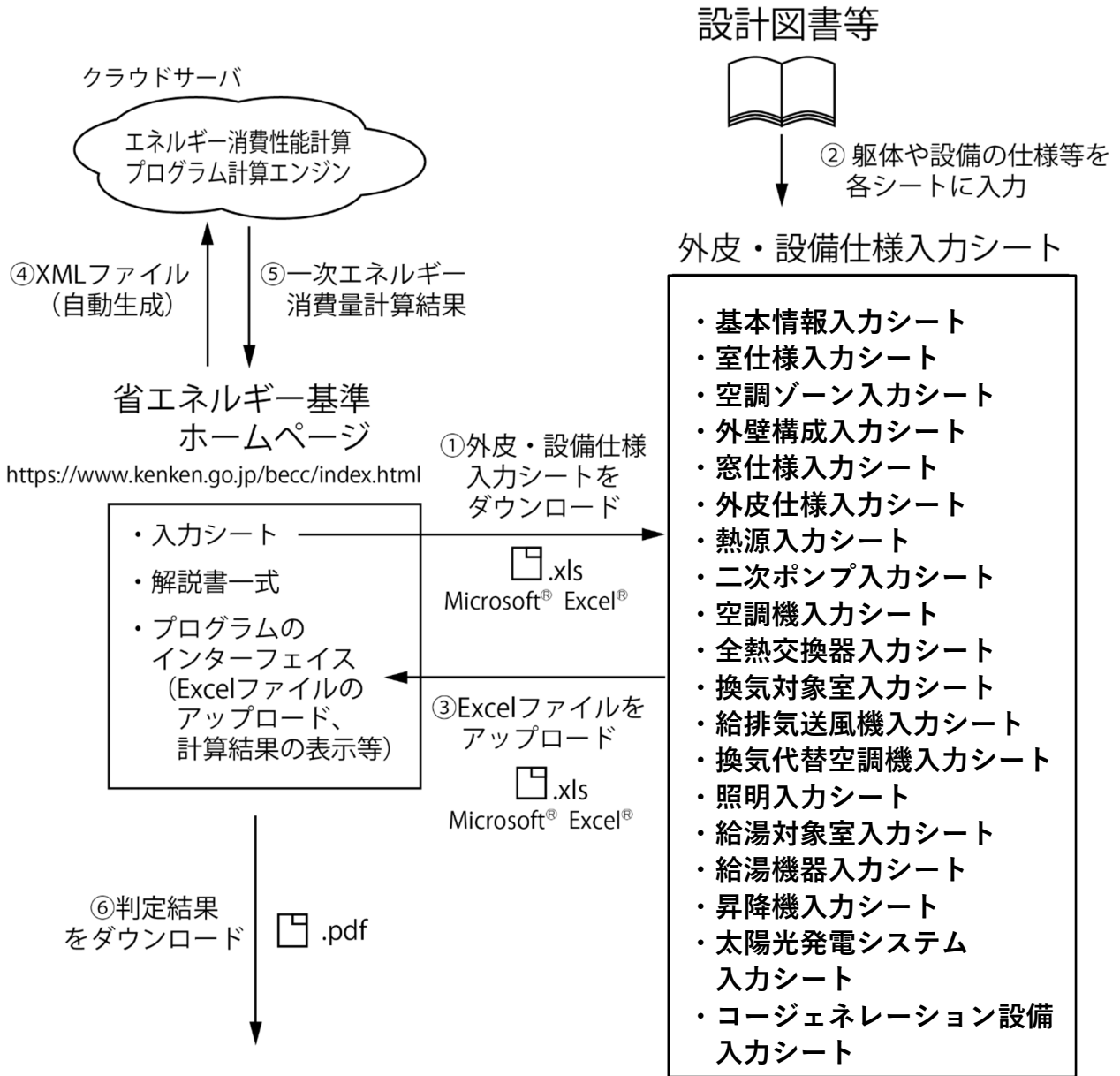
図 0-2-4 エネルギー消費性能計算プログラム（非住宅版）による評価の流れ
