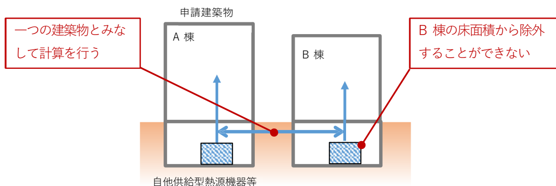
図 12-3-1 各建築物の熱源間で熱融通を行う場合
