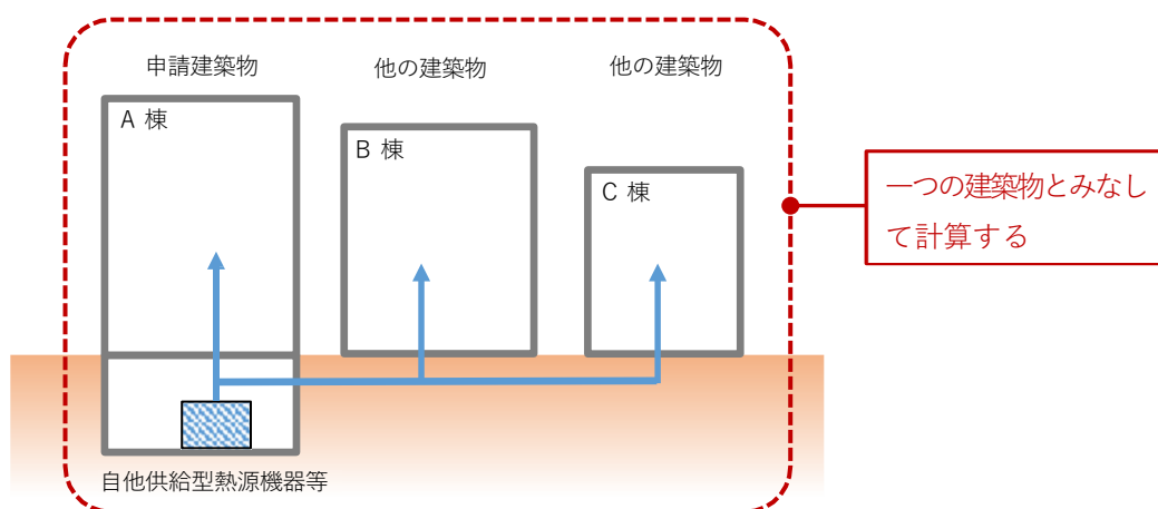
図 12-2-1 計算の基本的な考え方
