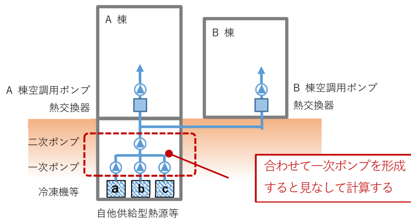
図 12-3-3 自他供給型熱源機器等が二次ポンプシステムの場合
